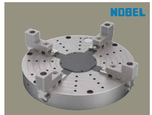
薄型軽量インデペンデントチャック TIシリーズ
